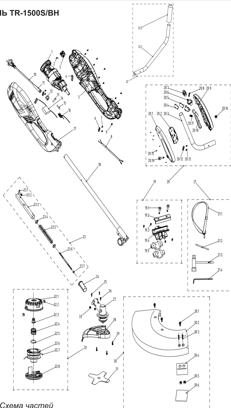
Рис. 6. Схема частей
